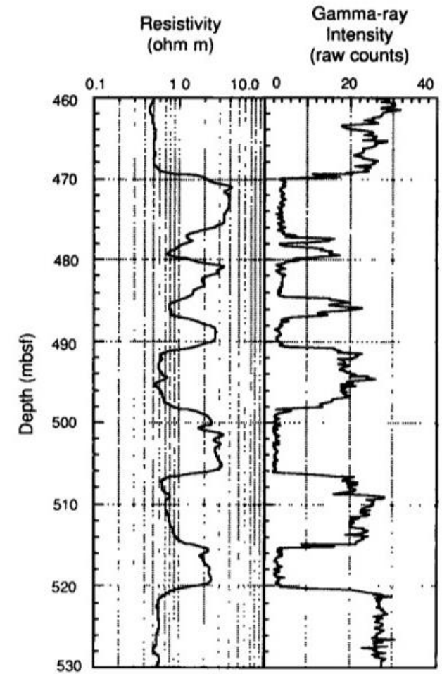
Hole 857C
