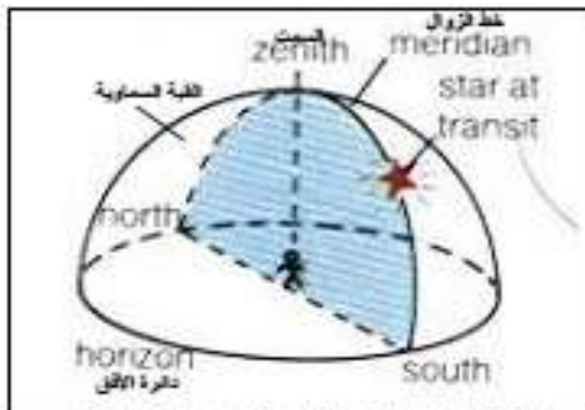
شكل ٣-٢ : الكرة السماوية، وتتألف فيها نقطة السميت، ودائرة الزوال والأفق.
