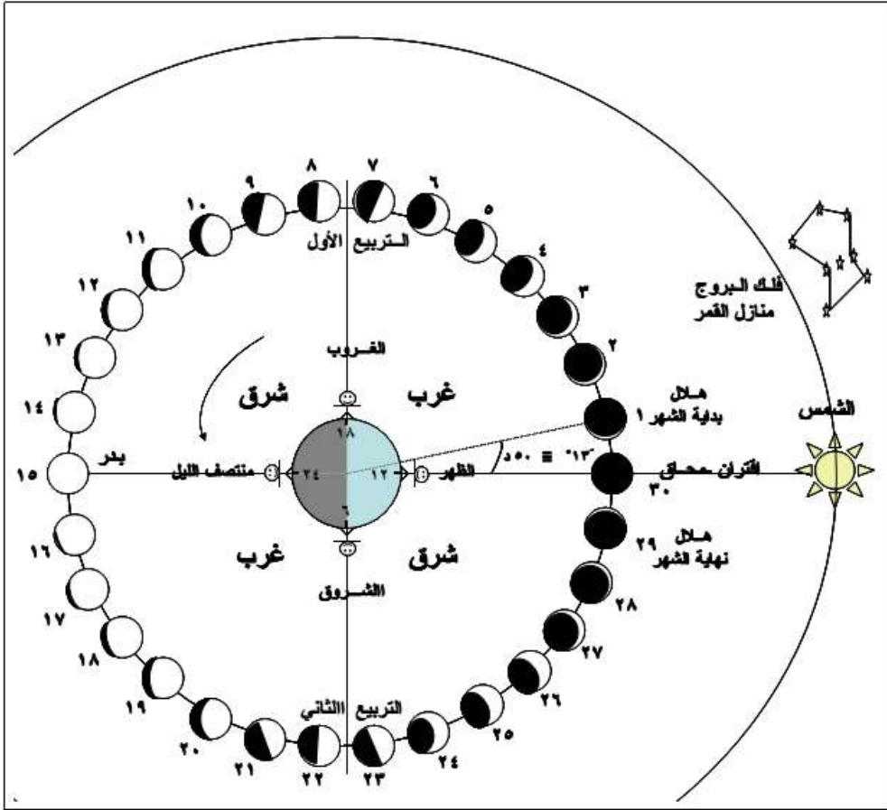
شكل ٢-٣: دورة القمر حول الأرض والشكل الظاهري لأطوار القمر
