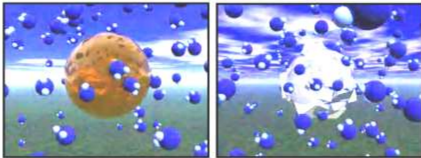
نويات تكثيف غير متميعة
