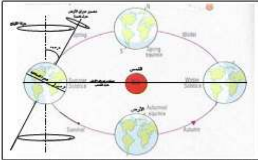
شكل ٣-٢ : حركات الأرض حيث تدور الأرض حول الشمس وحول نفسها وتتملك محوراً يميل حول المحور العمودي على مستوى دورانها حول الشمس أو على خط البروج (حركة التراجع).
