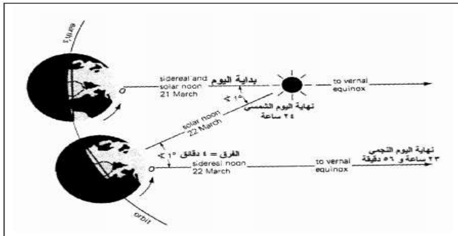
شكل ٨-١: الفرق بين اليوم النجمي واليوم الشمسي.
