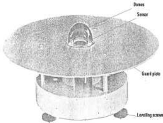
Pyranometer
