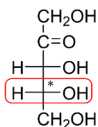
D-Ribulose
