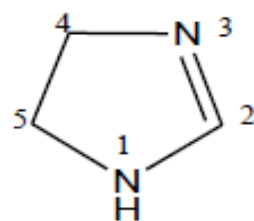
\Delta^2 -1,3-Diazoline
