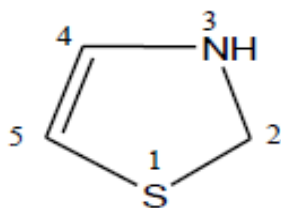
\Delta^4 -1,3-Thiazoline
