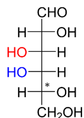
D-Galactose
