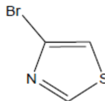
4 bromo 1,3 thiazole
