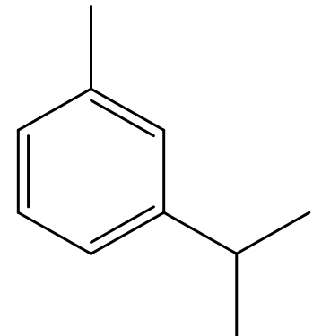
m-cymene
