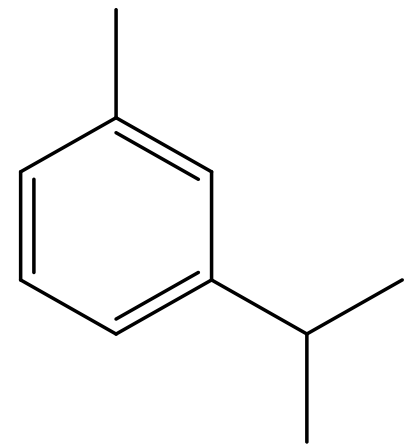
m-cymene
