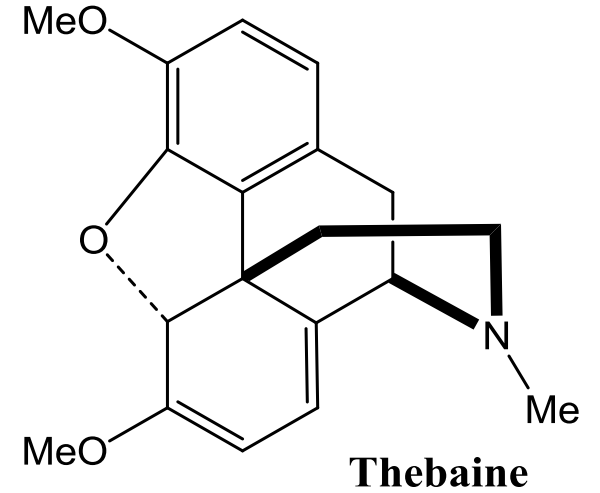
قلويد الثيبايين
