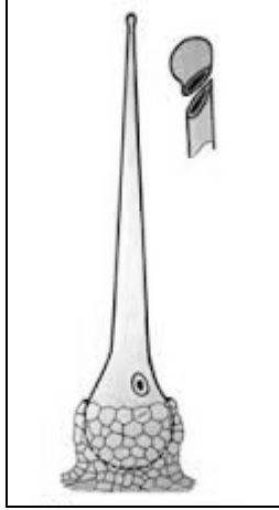
الشعيرة اللاسعة
