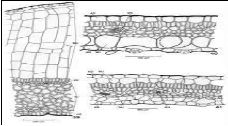
البشرة المركبة
