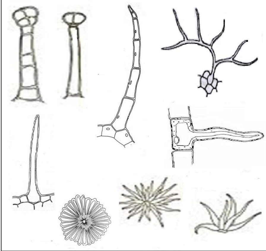
انواع الشعيرات
