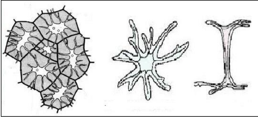
الخلايا الحجرية
