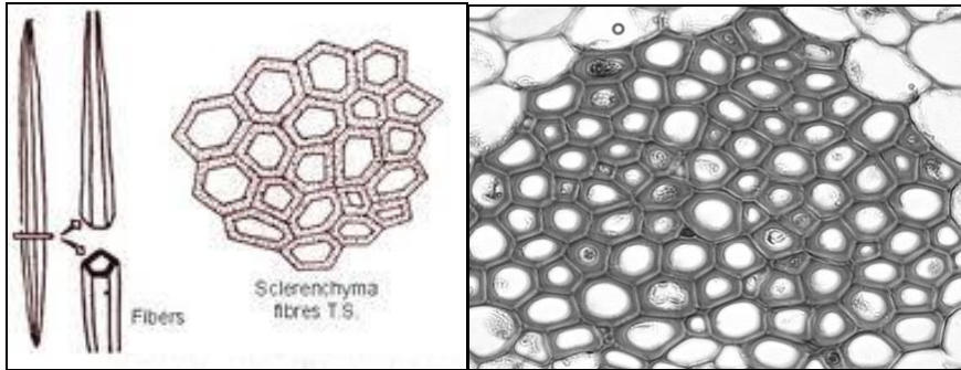
الألياف
