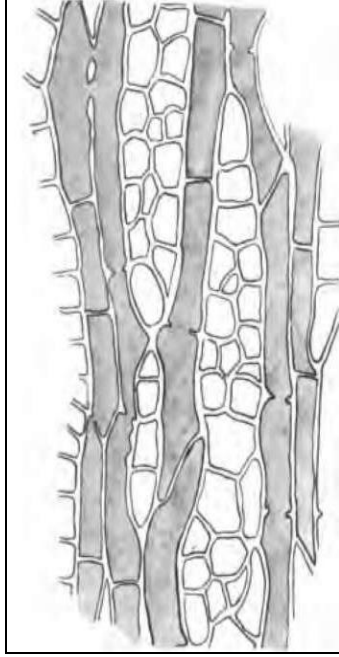
الاعية اللبنة
