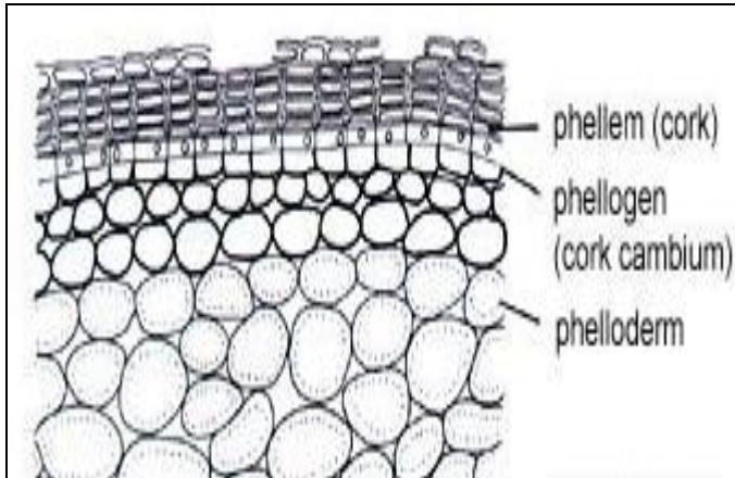
نسيج البريديرم
