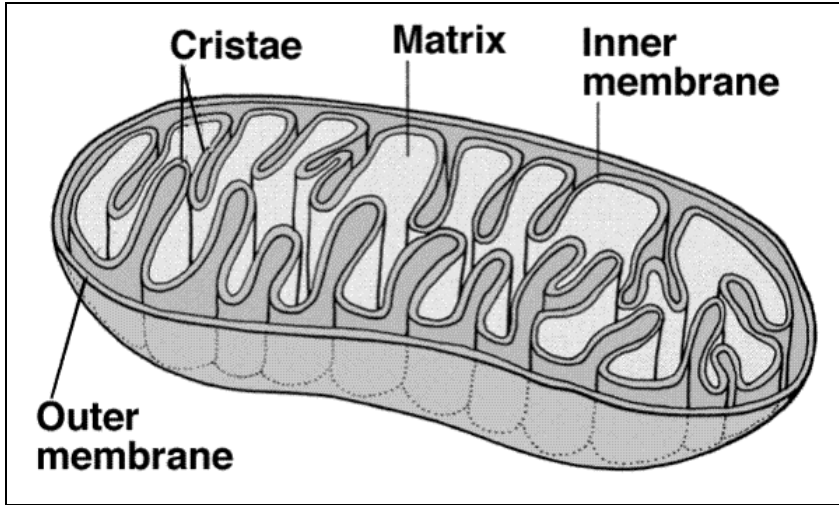
تركيب الميتوكوندريا
